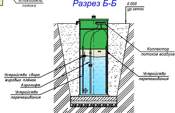
Разрез Б-Б
